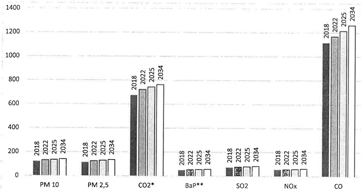
Wykres 8. Graficzne przedstawienie emisji zanieczyszczeń w ujęciu globalnym w gminie Koziernice wg scenariusza zaniechania w [Mg/rok].
