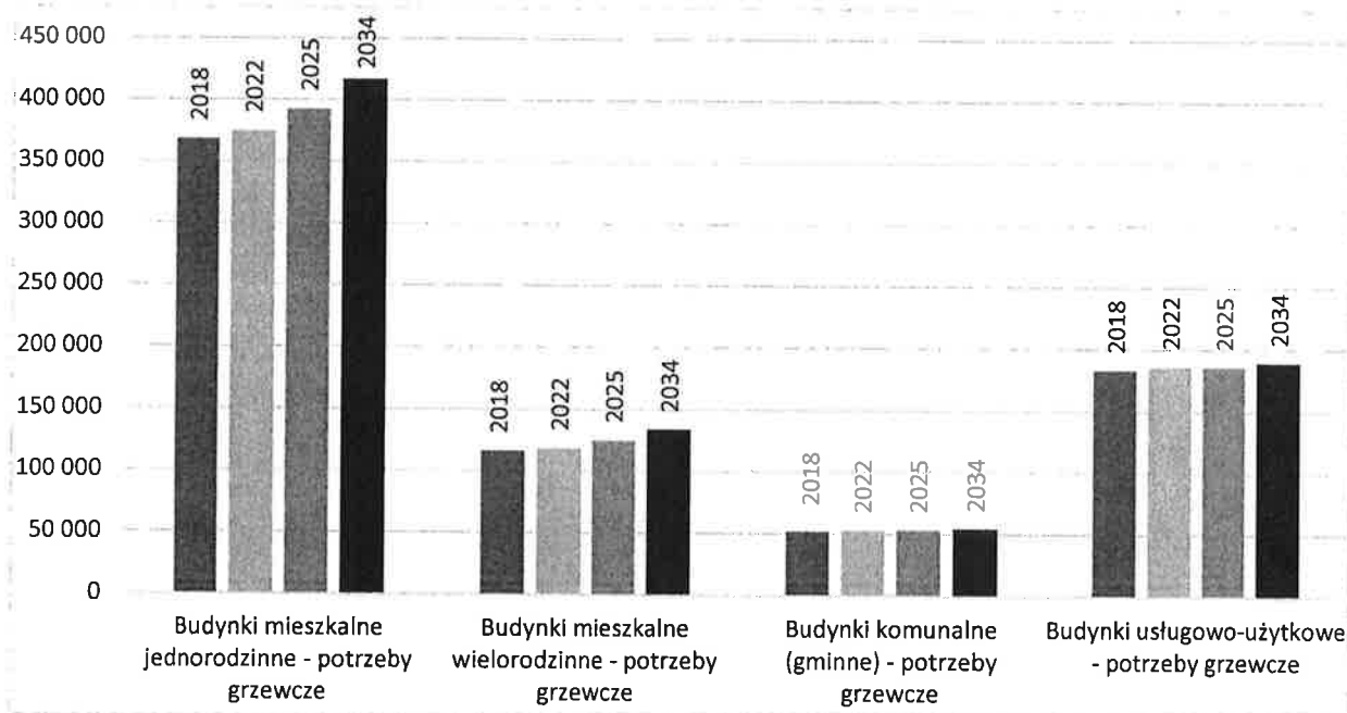
Wykres 6. Zużycie energii dla budownictwa na terenie Gminy Koziénice dla poszczególnych sektorów na potrzeby grzewcze, wg scenariusza zaniechania.
