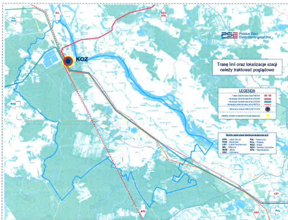
Rysunek 32. Schemat sieci przesyłowej na obszarze Gminy Kozienice - stan na 2032 rok źródło:[24]
